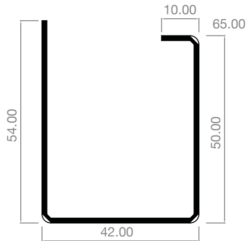
AE5349GS/6 (EWS618S) DOOR SASH
