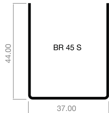
AE/BR45S bevel mid T & Z & ovolo T & Z & door sash T & Z
