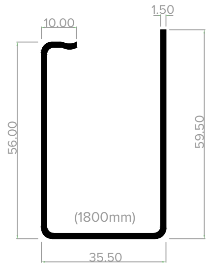
AE3660GS/HDI8 115mm T & Z DOOR SASH
